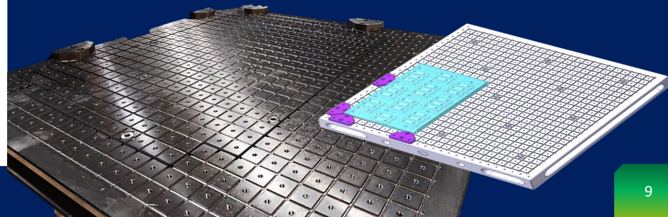
B) Kontúron változtatható 25×25 mm raszter-elosztás, amelyen csavarok állításával állíthatók a szívóhelyek
