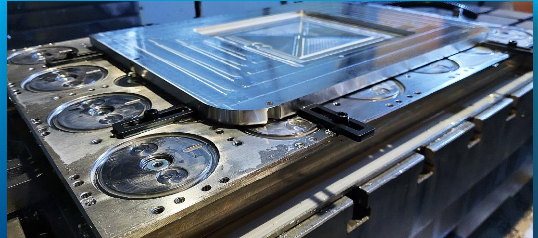
A) D75 mm korongok látják el a szívóerőt és az alátámasztást
